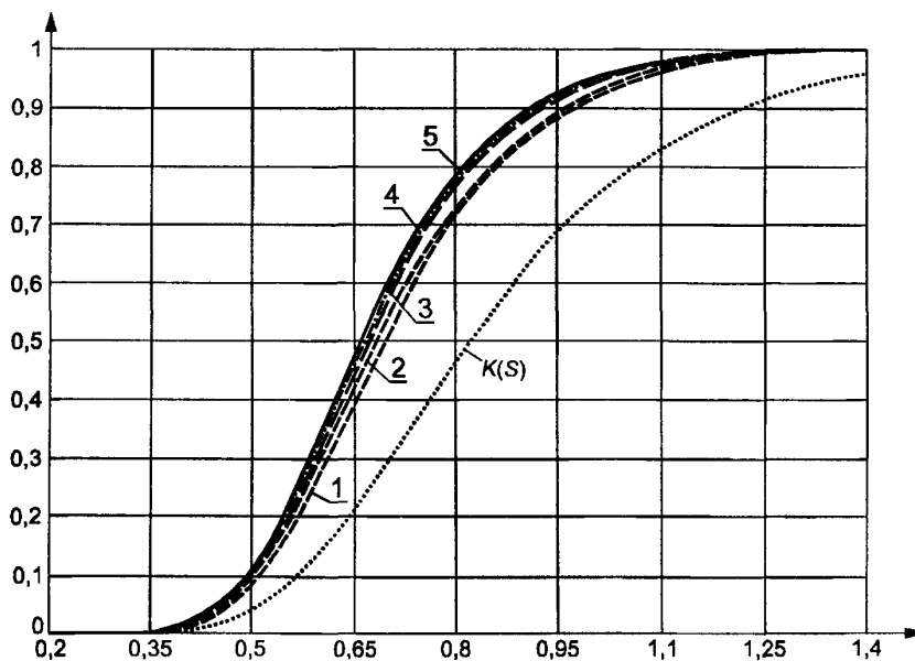
Рисунок 21 — Функции распределения статистики S_K Колмогорова при вычислении ОМП параметра формы гамма-распределения: K(S) — функция распределения Колмогорова
